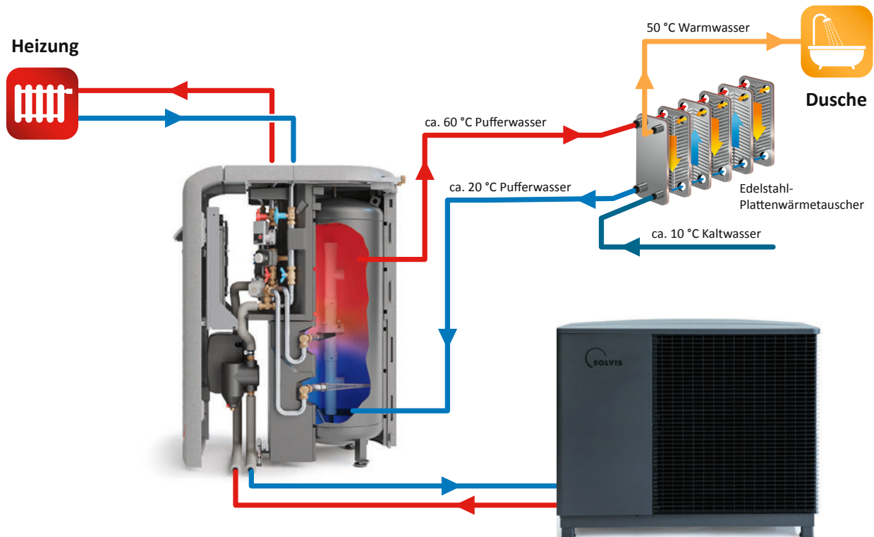
Heizkreislauf mit Wärmepumpe SolvisLea Pro und Pufferspeicher SolvisBen mit 230 l.
