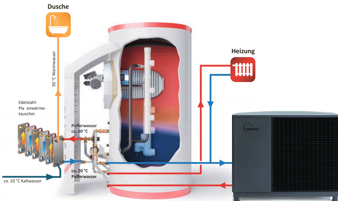
Alternativ SolvisMax mit noch größerem Wärmespeicher von bis zu 950 l Fassungsvermögen.
