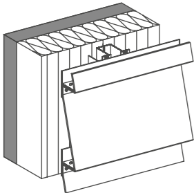
8 GENIETETE STÜLPSCHALUNG auf Aluminium-Unterkonstruktion
