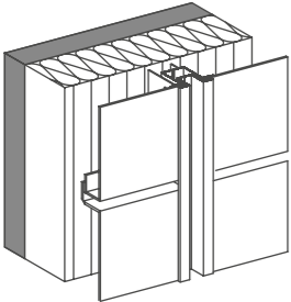
7 GEKLEMT/GESCHRAUBT auf Doppelhutprofilen
